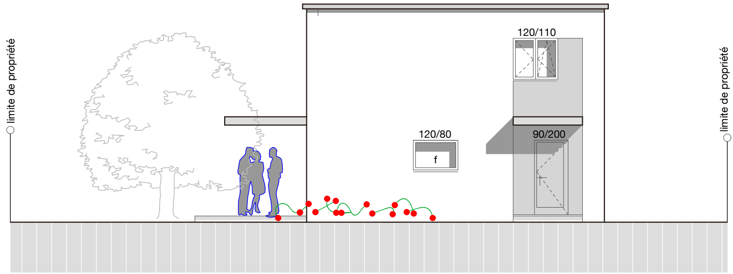
FACADE SUD EST A
